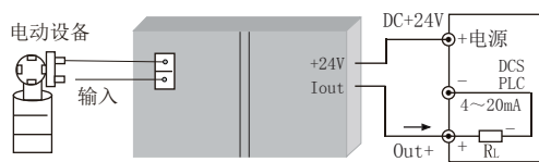
接线图二
