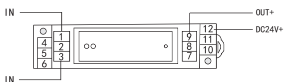
接线式
