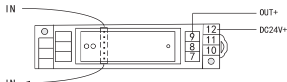
穿孔式
