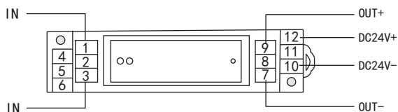
接线式
