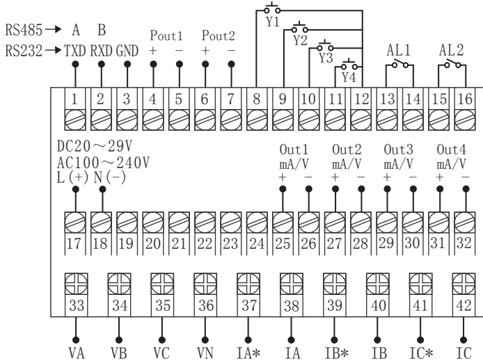
规格尺寸为S型接线图
