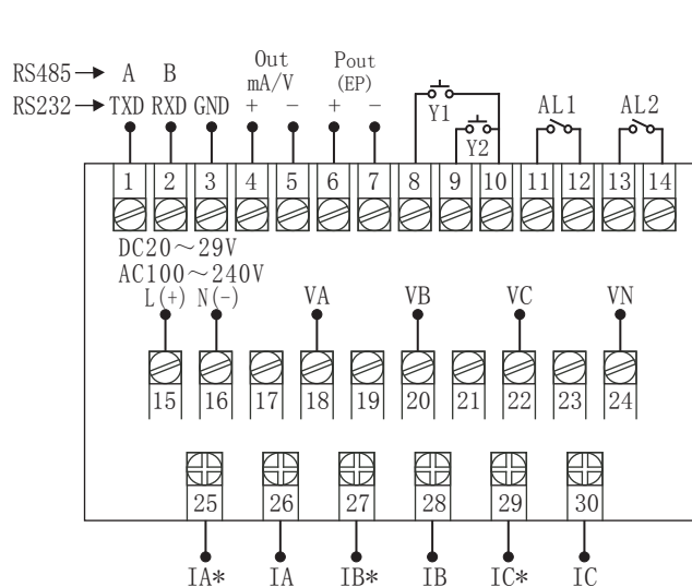
规格尺寸为R型接线图
